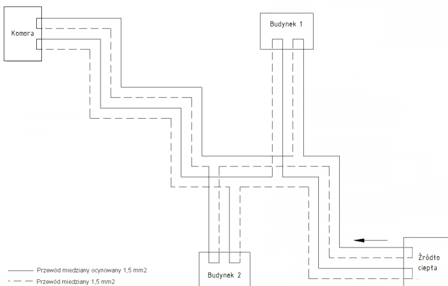
Rys.1. Sposób prowadzenia instalacji alarmowej
